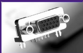
K61X 小型フットプリント 0.20" Footprint High Density Right Angle PCB Mount
